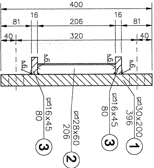
B-B 1:5
