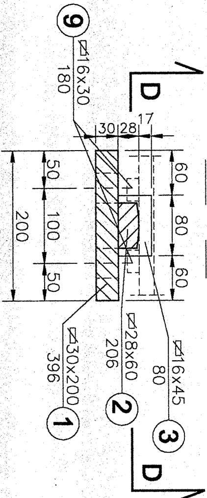
A-A 1:5
