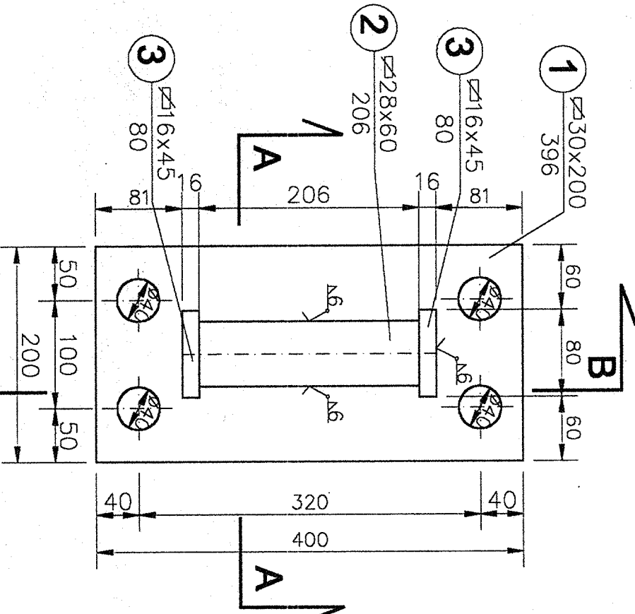
Widok z góry 1:5
