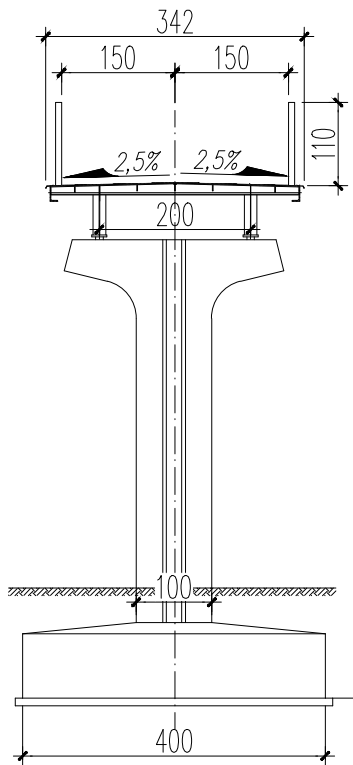
PRZEKROJ POPRZECZNY Skala 1:100
