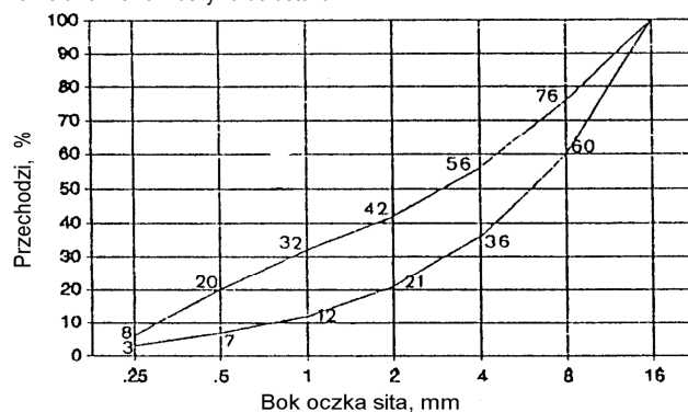
Rysunek 1. Krzywe graniczne uziarnienia kruszywa do betonu
