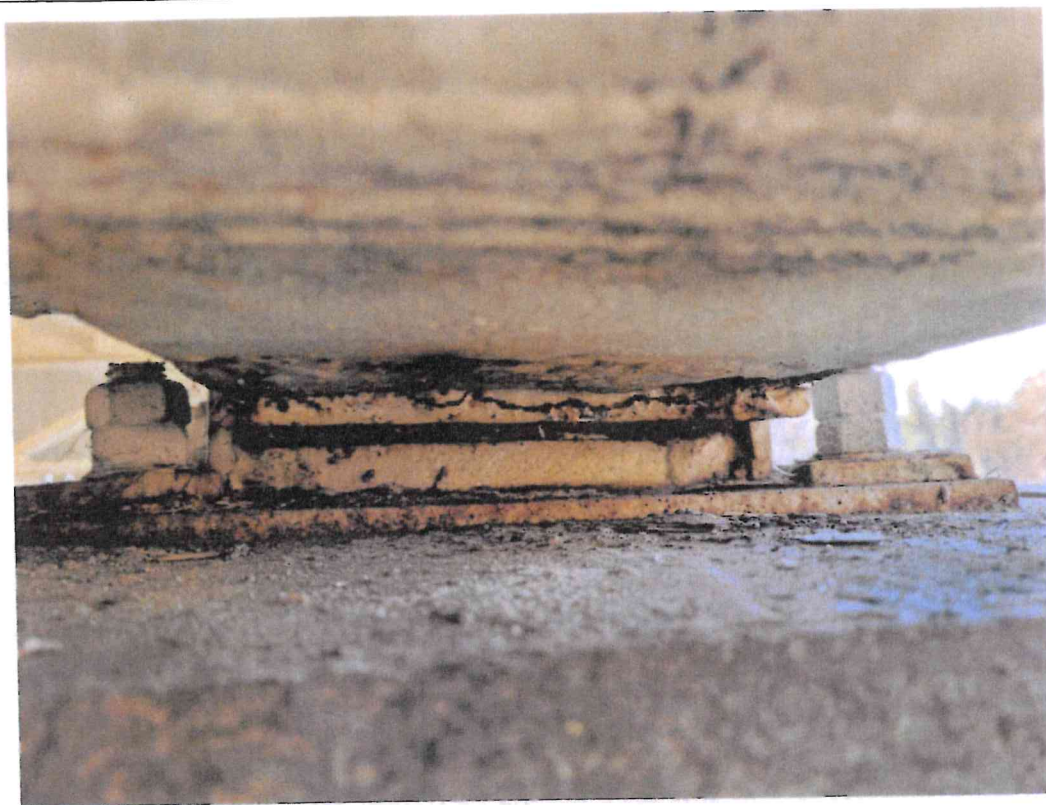
Fot. 13 Rozległa korozja łożyska. Pęknięcie spoiny łączącej łożysko z dźwigarem. Lokalizacja: Podpora północna, łożysko przęsła wiaduktu dla pieszych, przy schodach.
