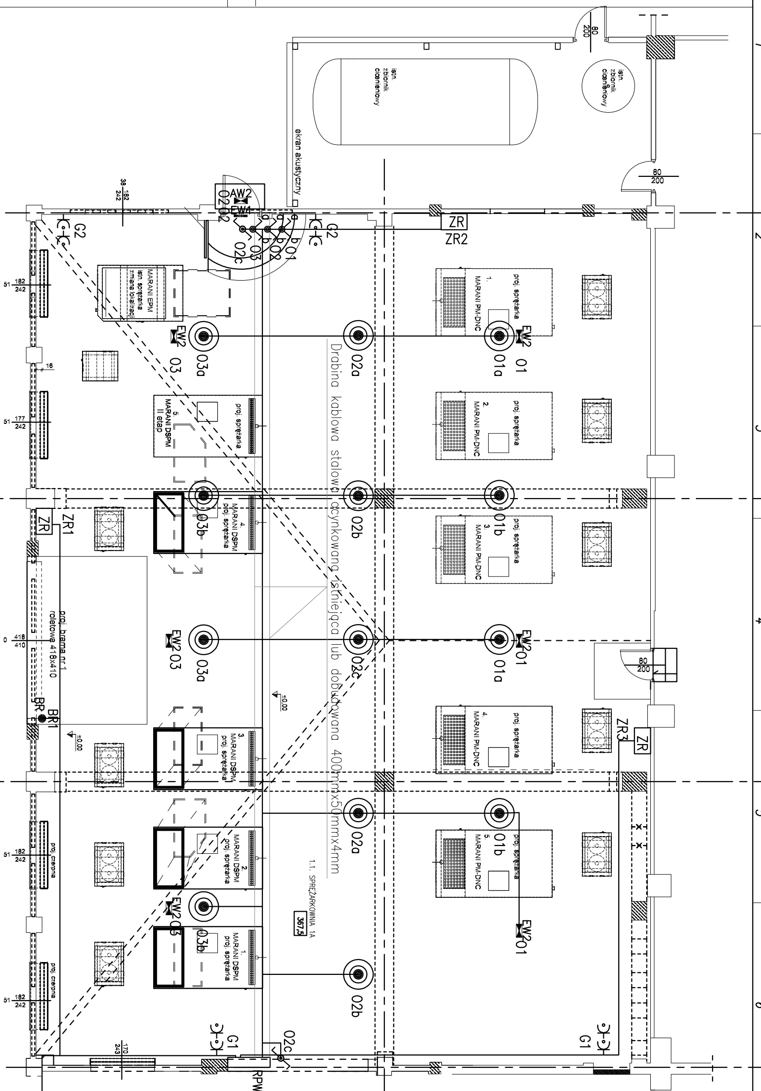
RZUT PARTERU
