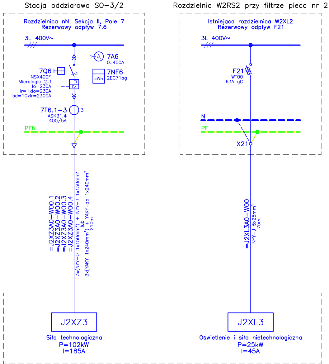
Projektowana rozdzielnia kontenerowa J2RS3 przy instalacji karbonatyzacji
