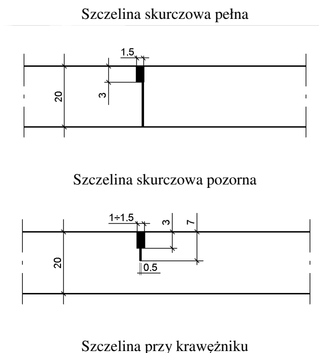
Rys. 1.1. Przykłady konstrukcji szczelin w podbudowie z betonu cementowego (wymiary w cm)
