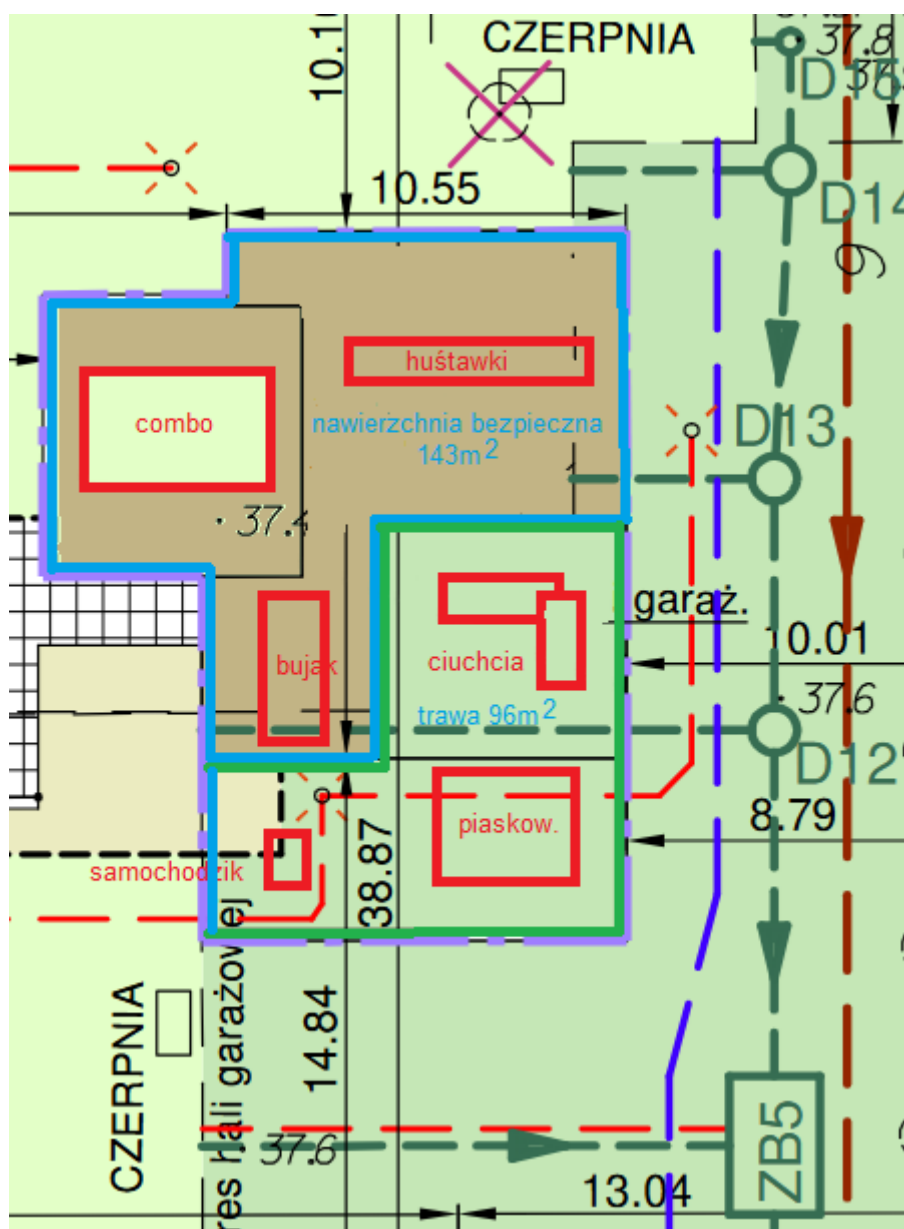
Schematyczne rozmieszczenie urządzeń oraz zakres nawierzchni
