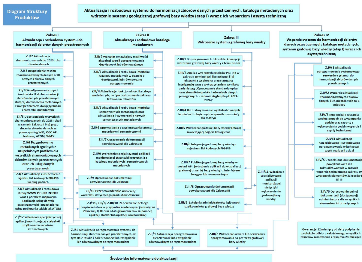
Rysunek 2. Diagram Struktury Produktów. Aktualizacja i rozbudowa systemu do harmonizacji zbiorów danych przestrzennych z uzupełnieniem zasobu zharmonizowanych danych, wdrożenie systemu geologicznej grafowej bazy wiedzy (etap I), aktualizacja i rozbudowa katalogu metadanych wraz z ich wsparciem i asystą techniczną. Rys. 2 jest również załącznikiem nr 2 Diagram Struktury Produktów do OPZ.
