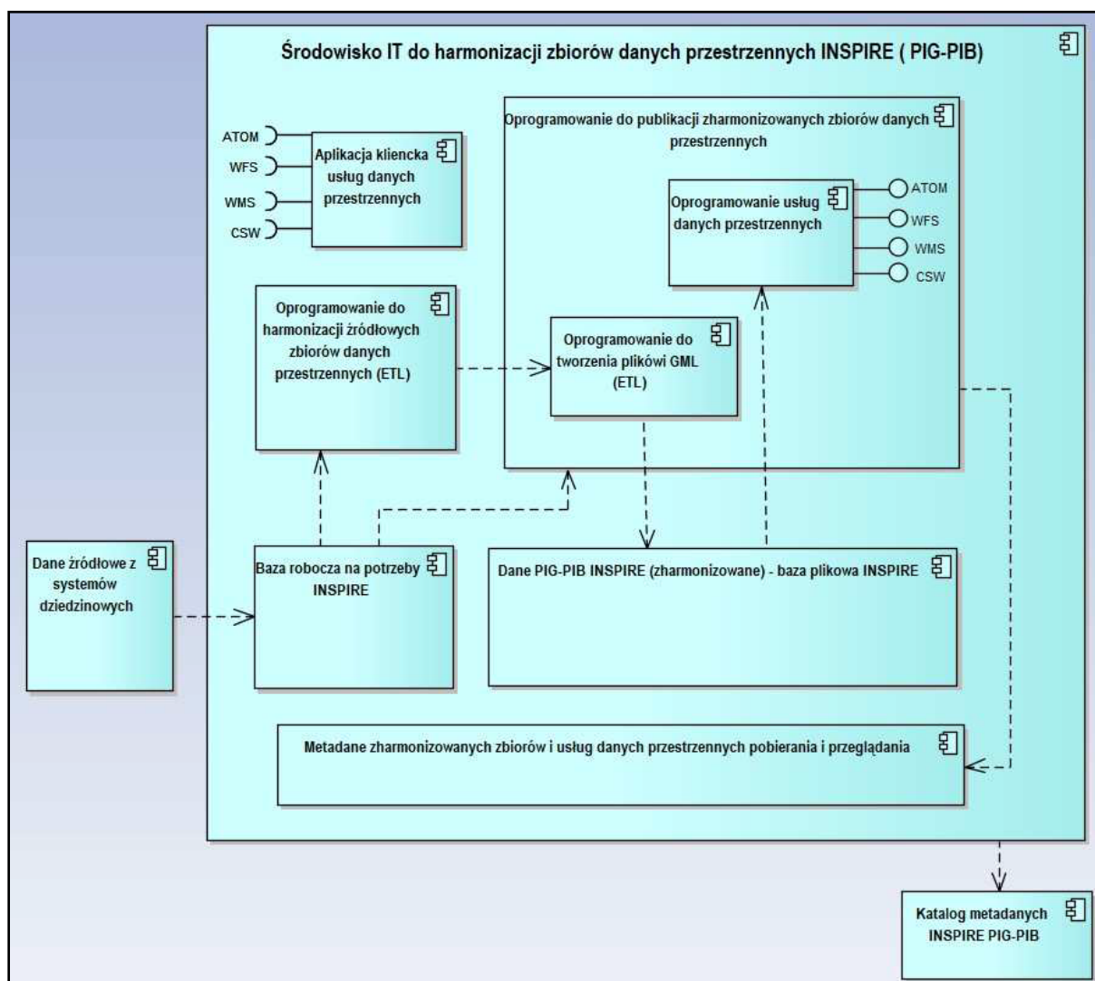
Rysunek 1. Aktualna architektura logiczna systemu do harmonizacji danych przestrzennych PIG-PIB na potrzeby INSPIRE.
