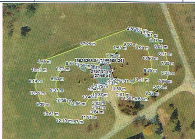
suw Zbiornik z obrysem powierzchni
