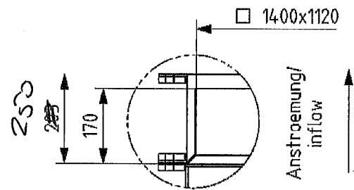
Detail U Massstab 1:10
