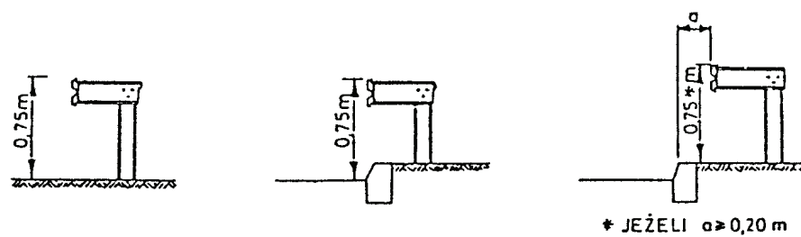
Załącznik 11.4. Profilowana taśma stalowa typu A i B, wg L. Mikołajków: Drogowe
